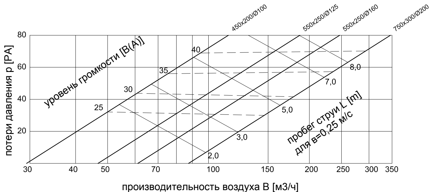
Вентиляционные головки NSCP/DZ с разжимным ящиком SR/NSCP
