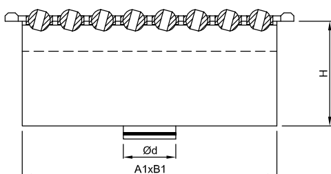
воздушный диффузор NSCP/DZ с разжимным ящиком SR/NSCP
