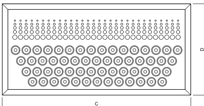
четыре ряда сопла
